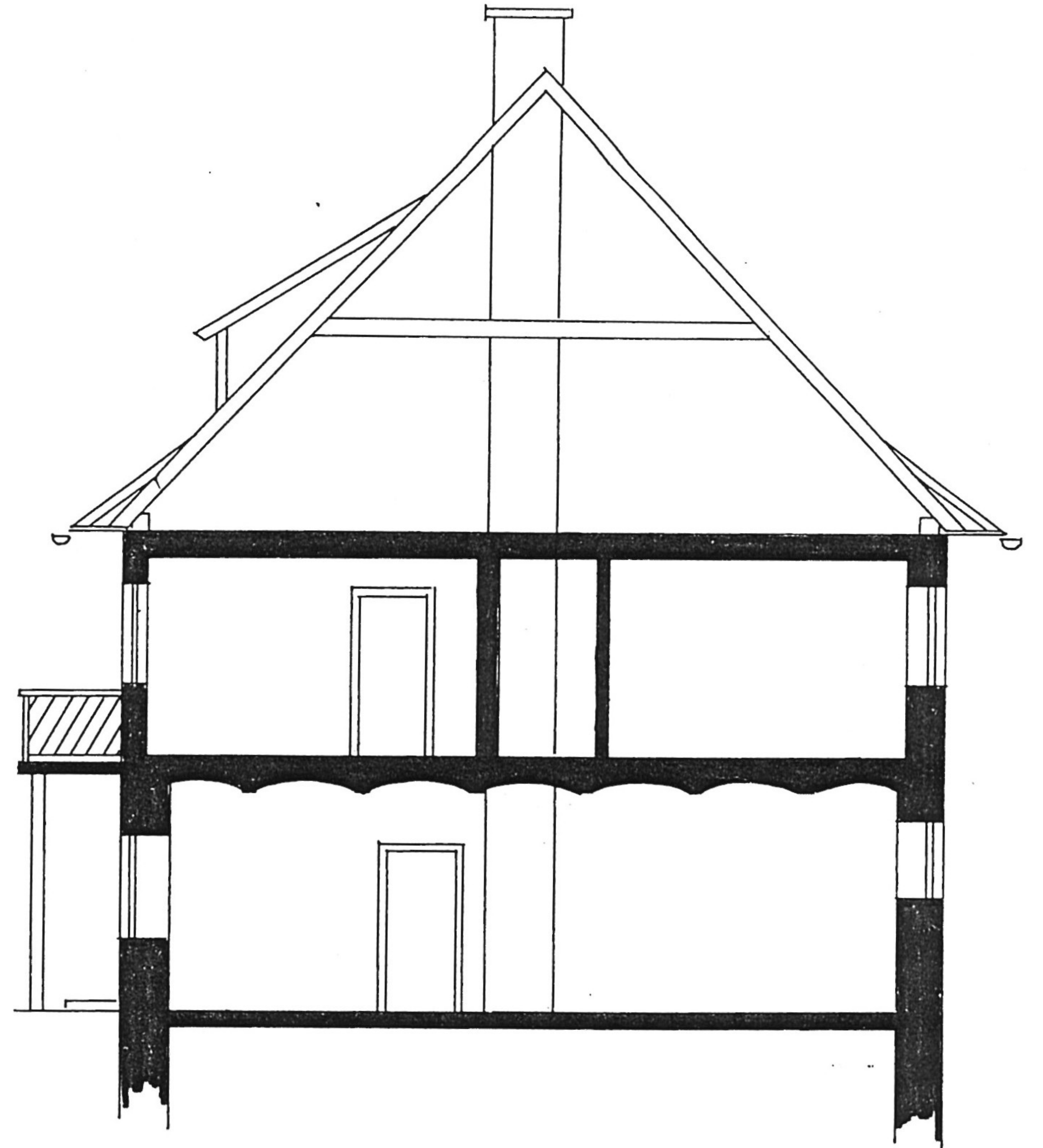
SCHNITT A - A
